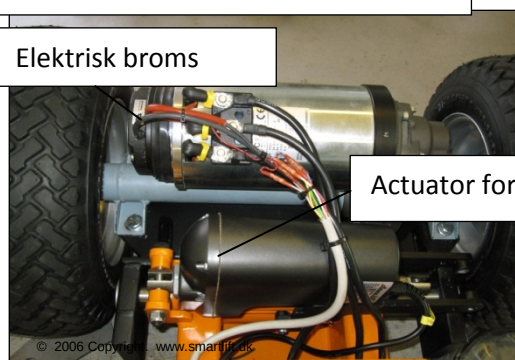
Framdrivningsmotor 1200 Watt AC. Drar på båda hjulen
