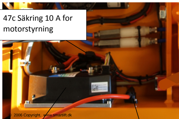
Motorstyrningsboks for AC-motor
