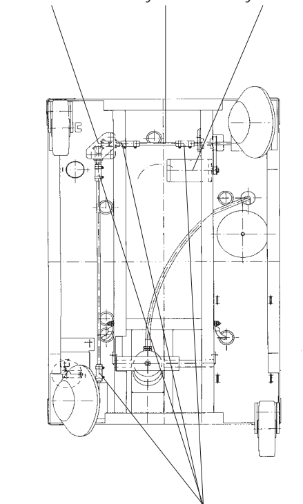
Öppningsbara axelkopplingar
